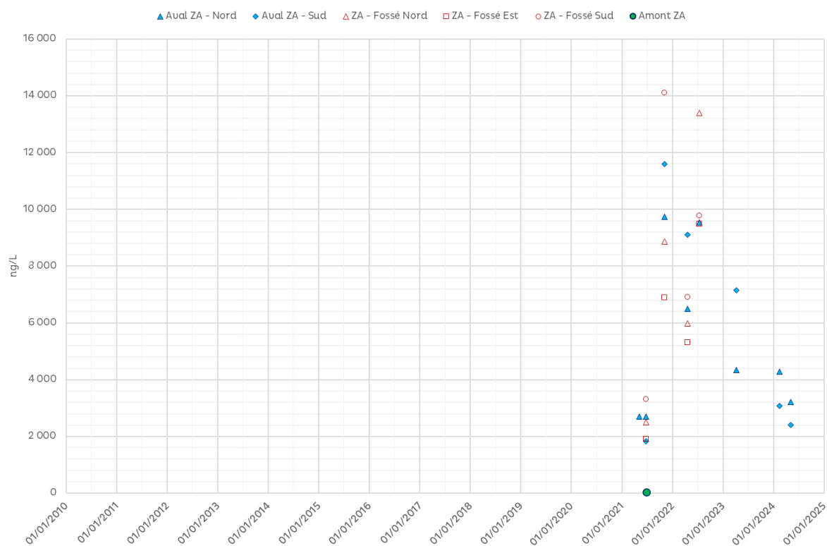
Figure 17 : Suivi des concentrations en métolachlore-ESA au niveau de la zone agricole de Blagon.
