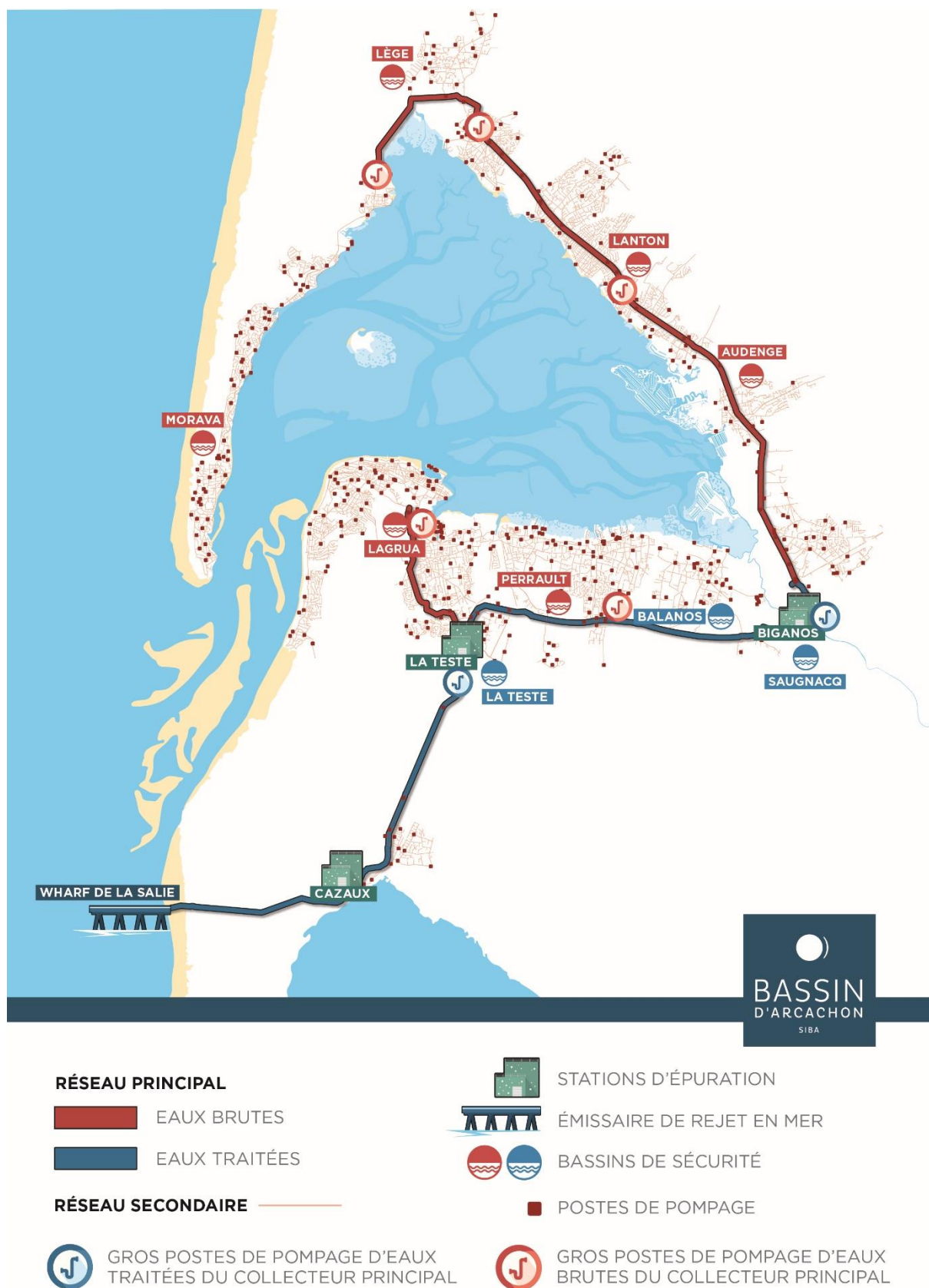
Figure 2 : Système d'assainissement des eaux usées des 10 communes riveraines du Bassin d'Arcachon
